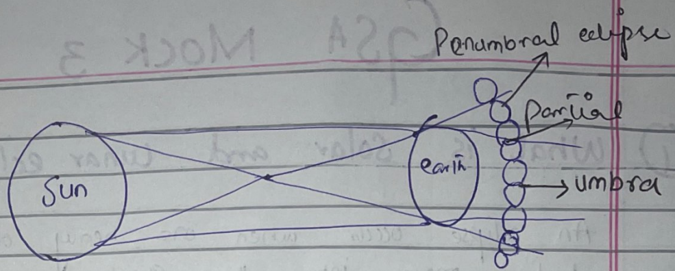
Lunar eclipse.
