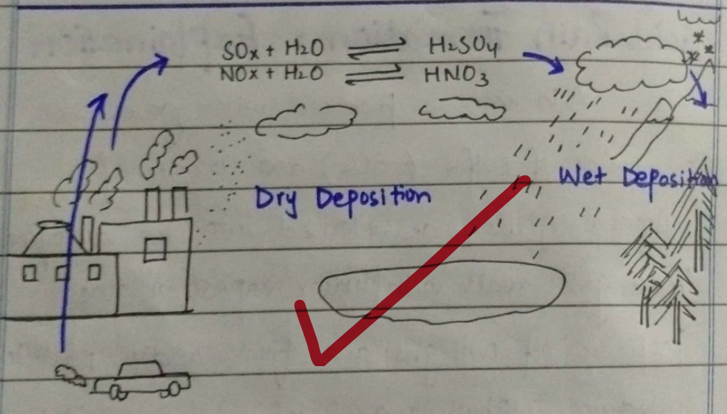
Fig 1 : Acid Rain
